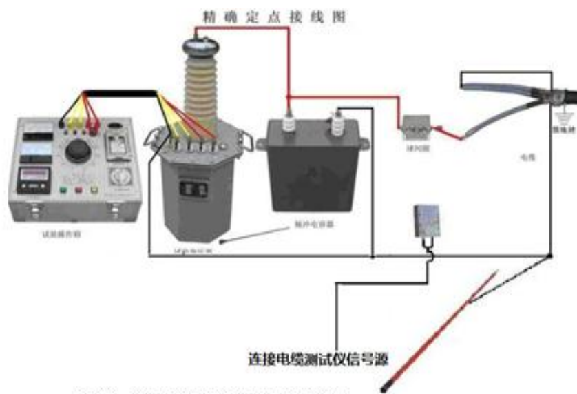
分体式高压测试实物连线图
