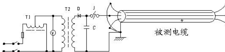
图9. 冲闪法放电接线图
